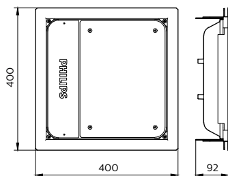
BBP500 G2 LED140/CW PSU A-WB
