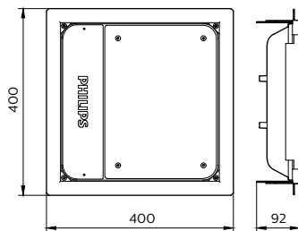
BBP500 G2 LED140/NW PSU A-WB
