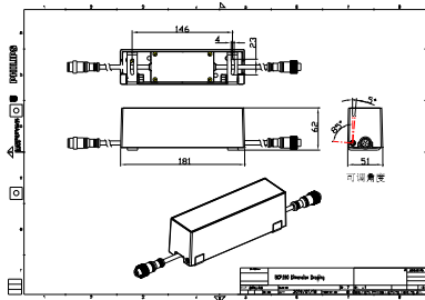
BCP390 3LED RGB 24V 3x90 DMX D3
