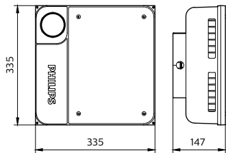
BCP500 G2 LED180/NW PSU S-WB
