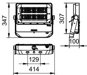
BVP432 LED269/CW 220~240V 200W AMB GM
