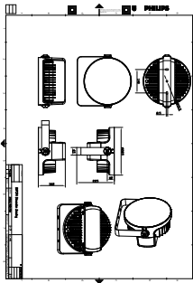
BVP374 48LED RGBNW 220V 60 DMX 120W HP
